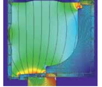
İzoterm çizgileri
